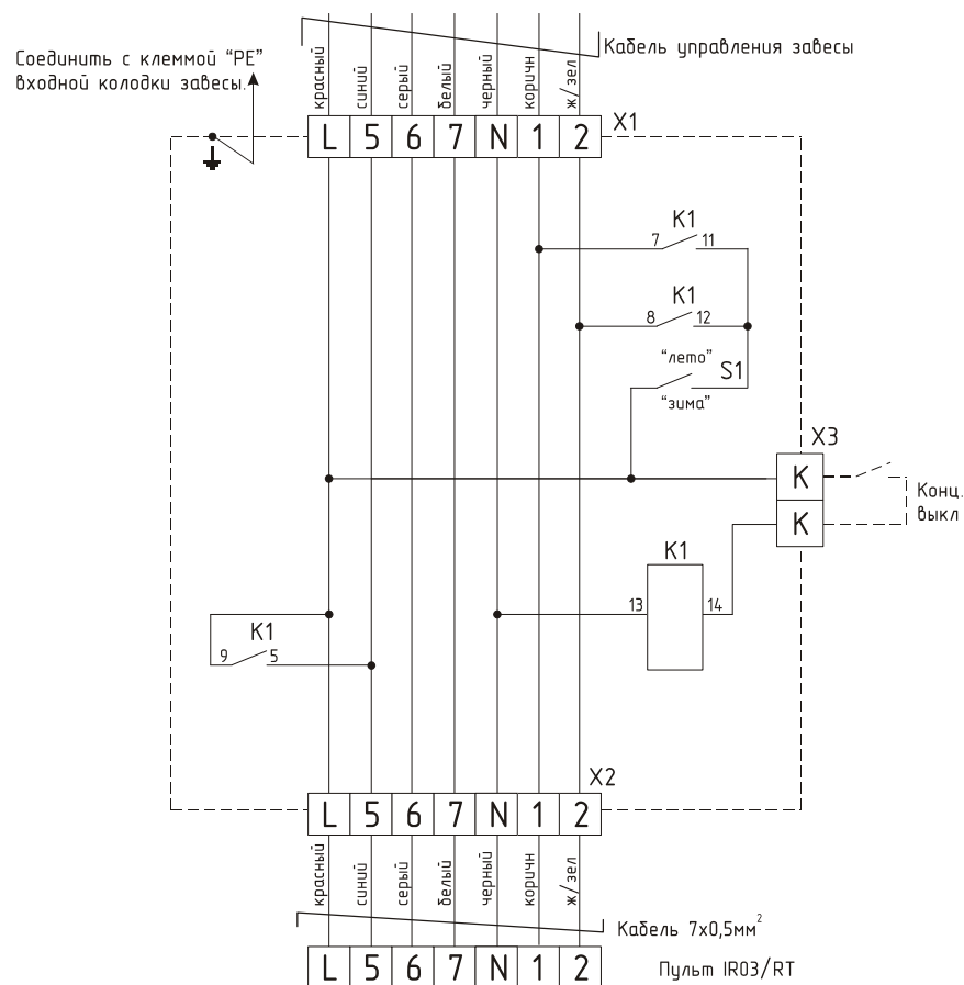
Рис. 10. Электрическая схема Блока подключения концевых выключателей к занесам с электрическим источником тепла.
