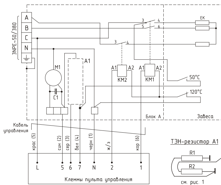
Рис. 3. Электрическая схема КЭВ-9П3030Е
