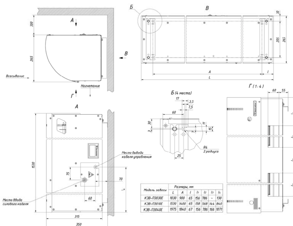
Рис. 11. Крепежные и габаритные размеры занес
